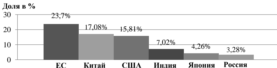
Рис. 3. Доля ВВП стран в мировом ВВП
