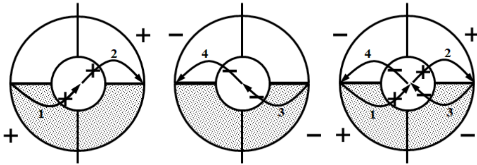
Рис. 3. Движение магнитных потоков Земли
