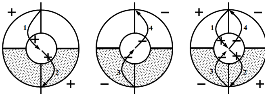
Рис. 2. Движение электрических потоков Земли
